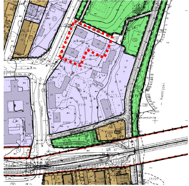
Kuva 4. Ote voimassa olevasta asemakaavasta. Suunnittelualue rajattu punaisella katkoviivalla.
